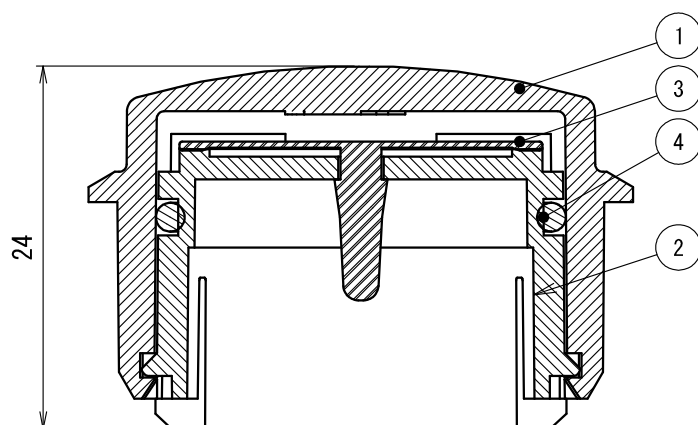
断面 A-A
